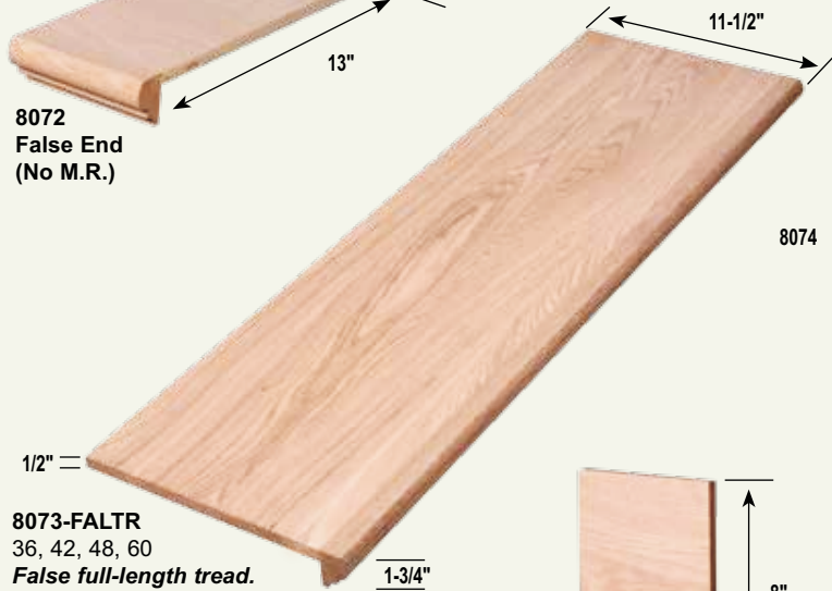
M.R. False End Specify: RH or LH
